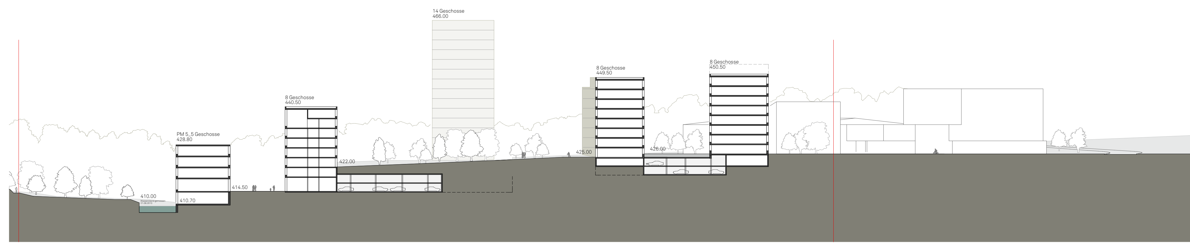
SCHNITT D-D M 1:750
